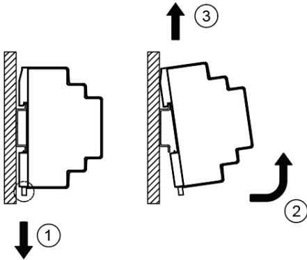
图. 2.2 拆卸
