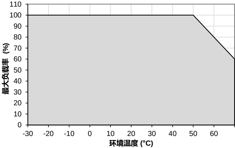
图. 1 垂直安装功率降额 > 50°C 功率降额 2.0% / °C
