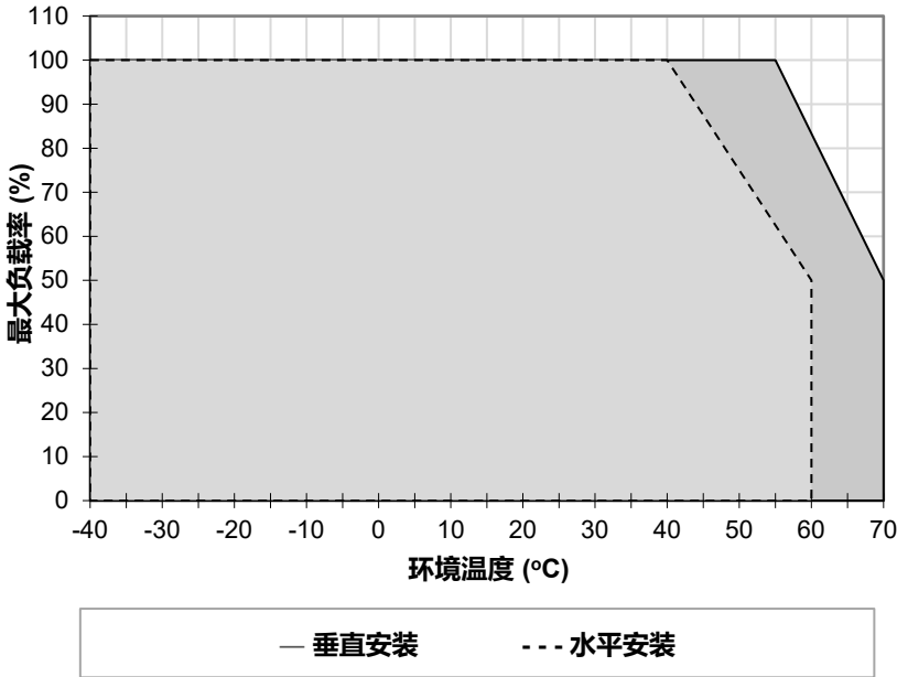
输出负载降额对应环境温度
