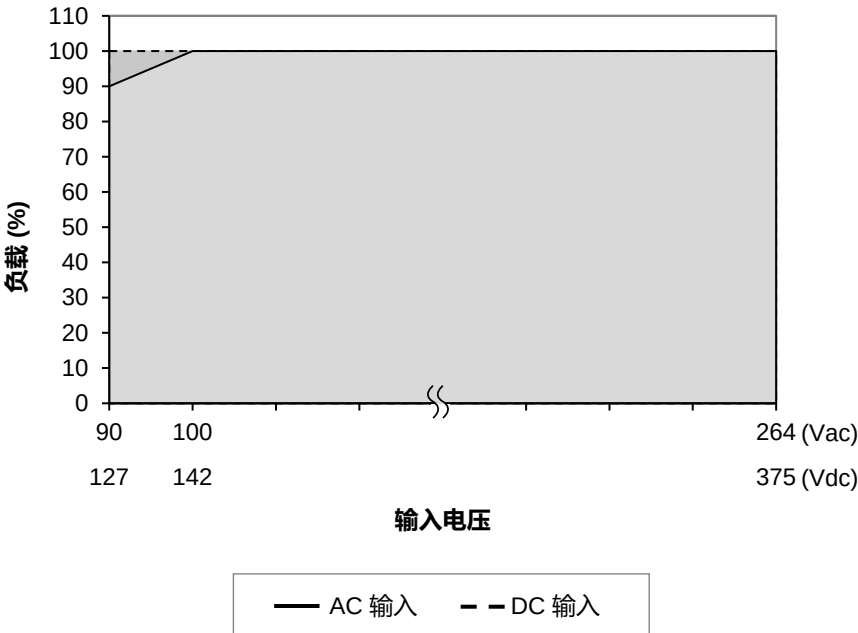
图. 2 AC & DC 输入电压功率降额 < 100 Vac 功率降额 1 % / Vac DC 输入无输出功率降额
