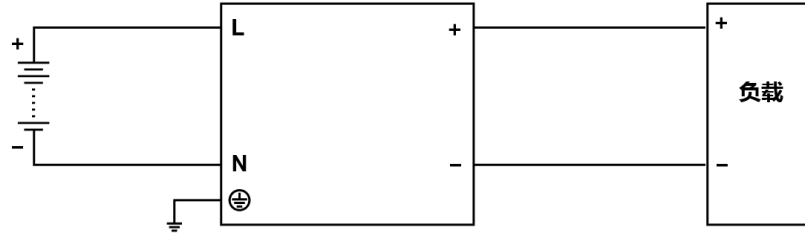
图. 4 DC 输入接线示意图
