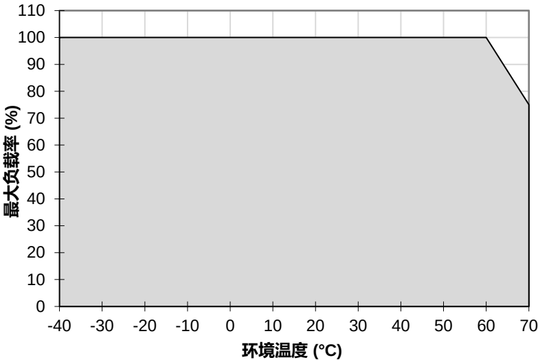
图. 1 垂直安装功率降额 > 60°C 功率降额 2.5% / °C
